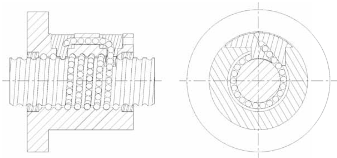
Fig. 3.24 V-type nut
