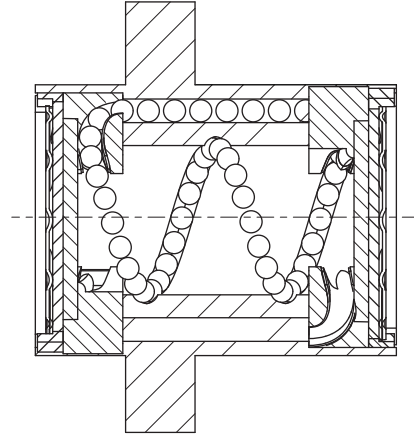
Fig. 3.25 Y- type nut
