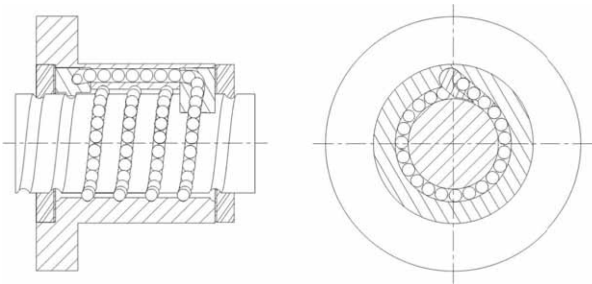
Fig. 3.23 S-type nut
